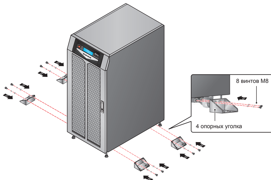
Рис. 6-4. Монтаж опорных уголков
