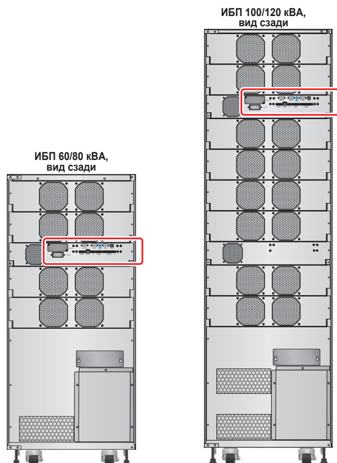
Рис. 5-1. Расположение коммуникационных интерфейсов
