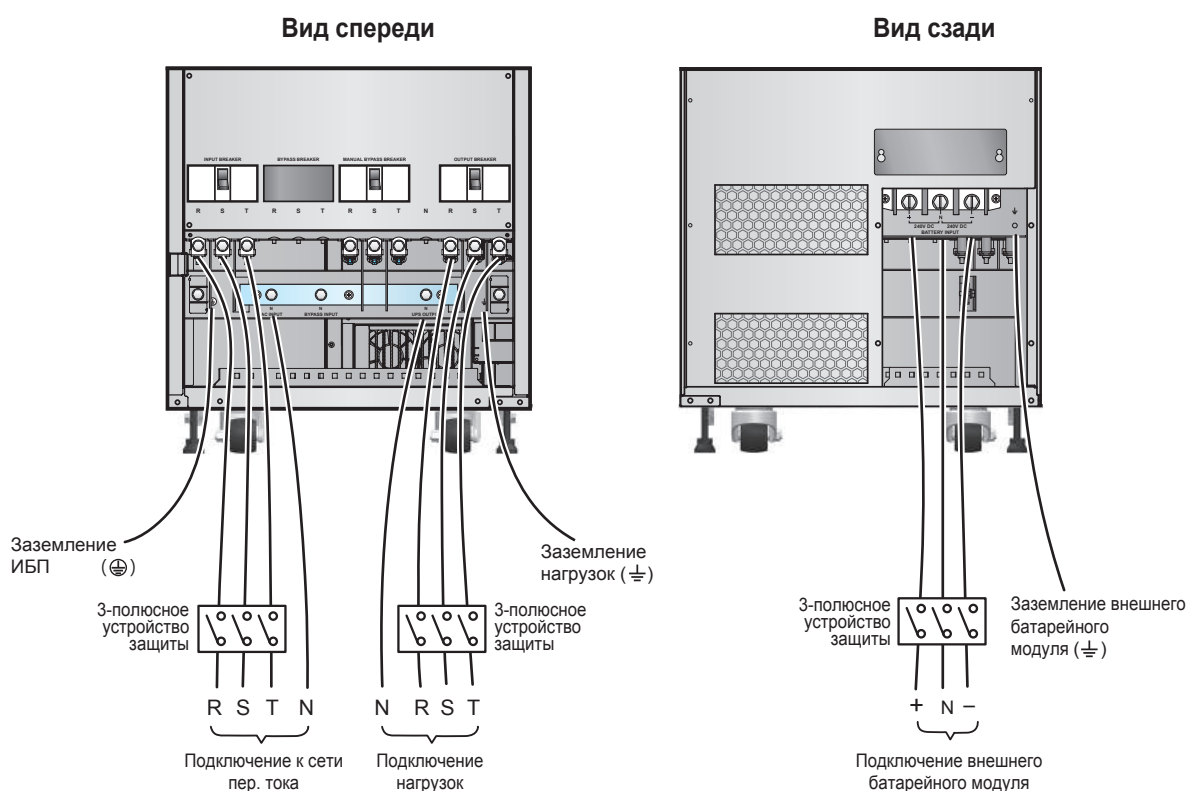
Рис. 6-11. Схема подключения одиночного ИБП 100/120 кВА в конфигурации с одним входом
