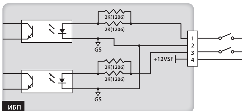
Рис. 5-7. Входы с сухими контактами, конфигурация I
