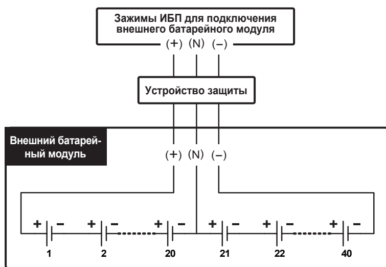
Рис. 6-17. Подключение внешнего батарейного модуля
