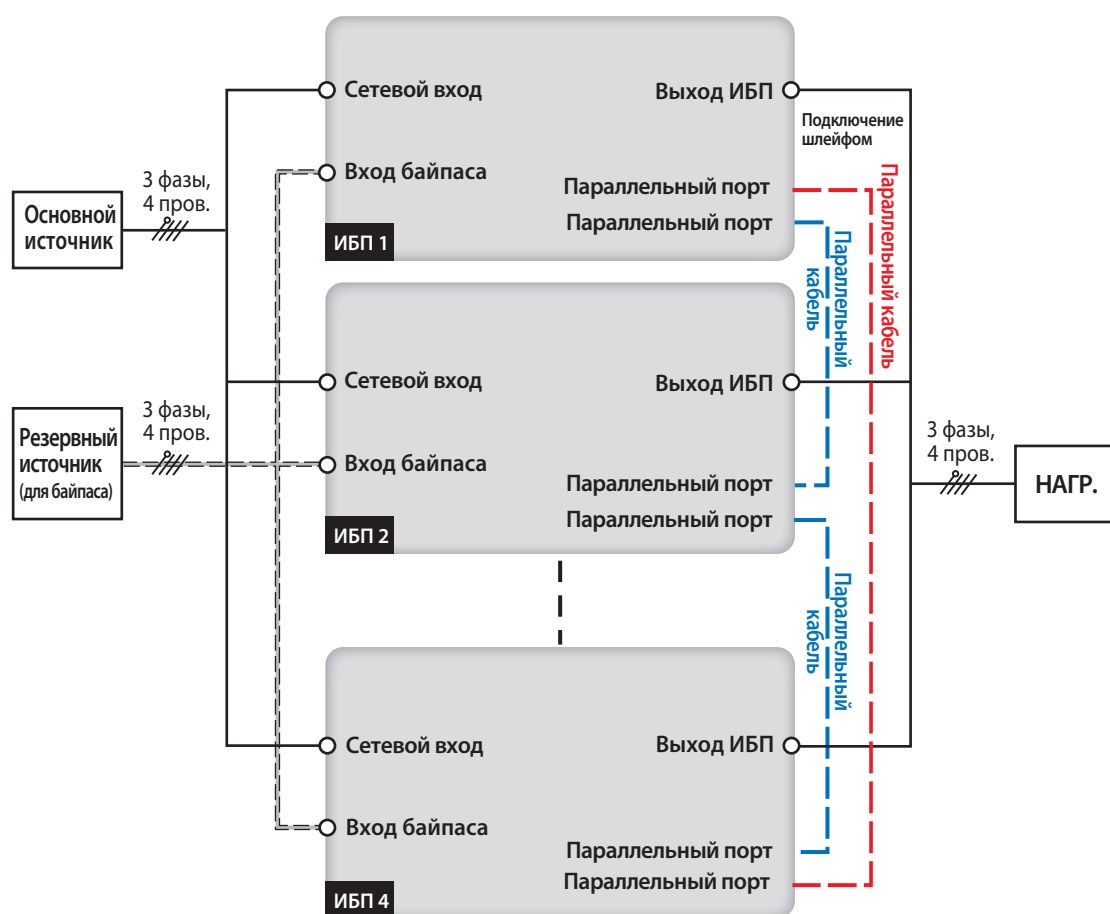
Рис. 6-16. Схема подключения в конфигурации с двумя входами (параллельные ИБП)
