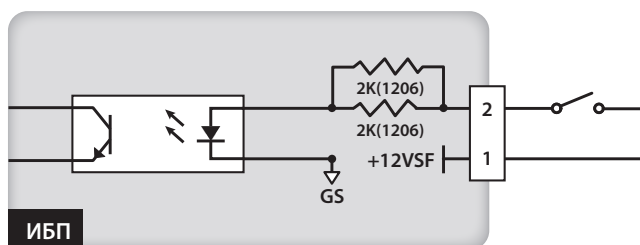
Рис. 5-5. Конфигурация порта REPO
