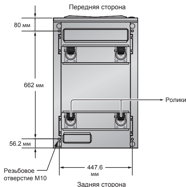
Рис. 6-2. Расположение крепежных отверстий
