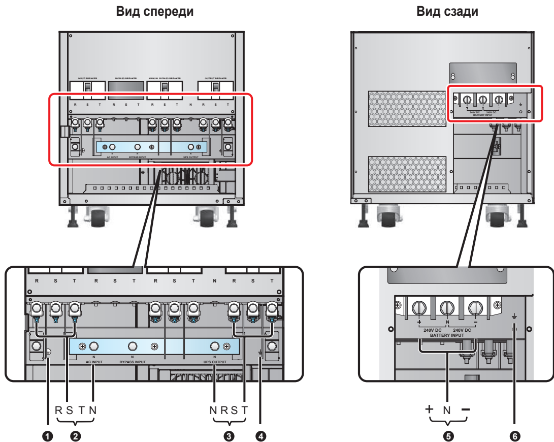
Рис. 6-8. Модель 100/120 кВА, блок зажимов
