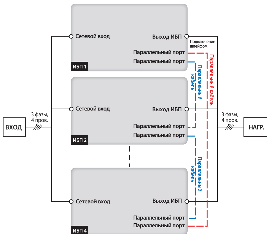
Рис. 6-15. Схема с двумя входами (параллельные ИБП)
