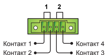
Рис. 5-6. Входы с сухими контактами
