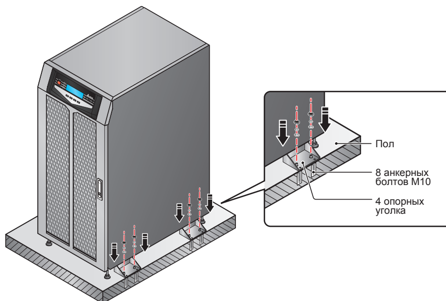
Рис. 6-5. Крепление опорных уголков к полу
