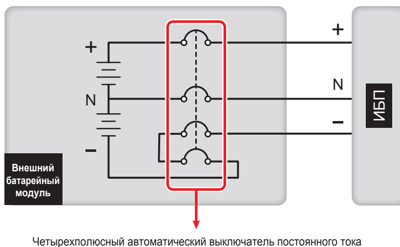
Рис. 6-19. Установка четырехполюсного автоматического выключателя постоянного тока
