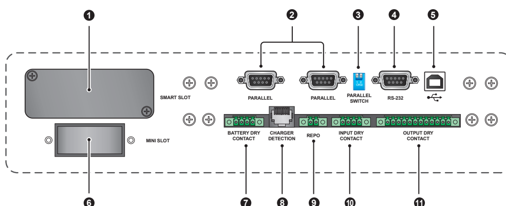
Рис. 5-2. Коммуникационные интерфейсы
