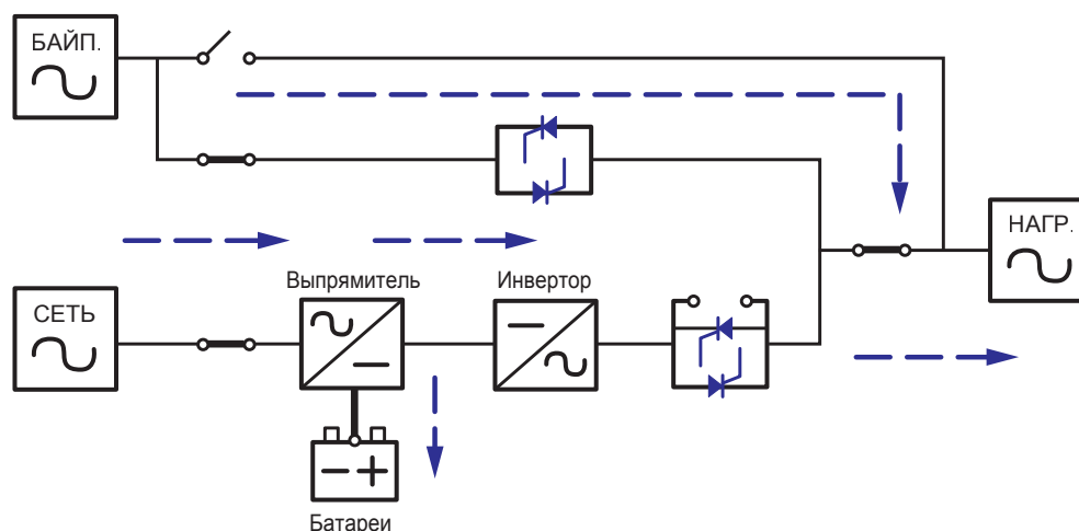
Рис. 4-3. Передача электроэнергии через ИБП в режиме готовности
