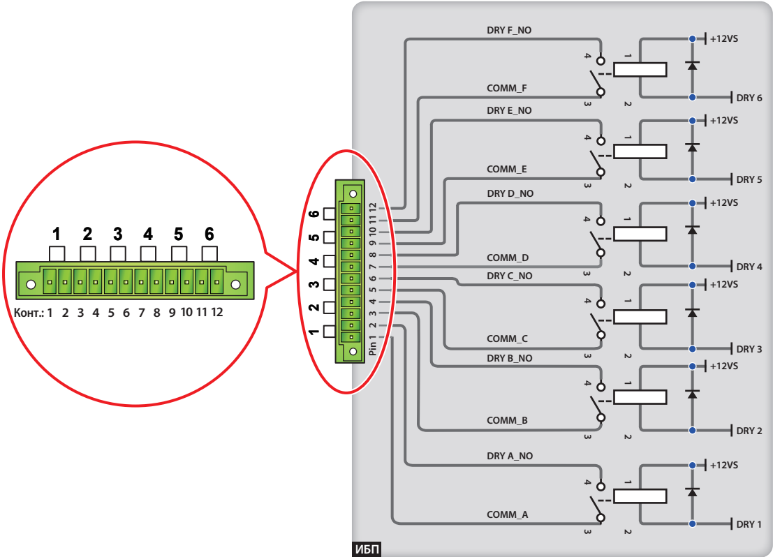
Рис. 5-9. Выходы с сухими контактами: назначение и подключение выводов
