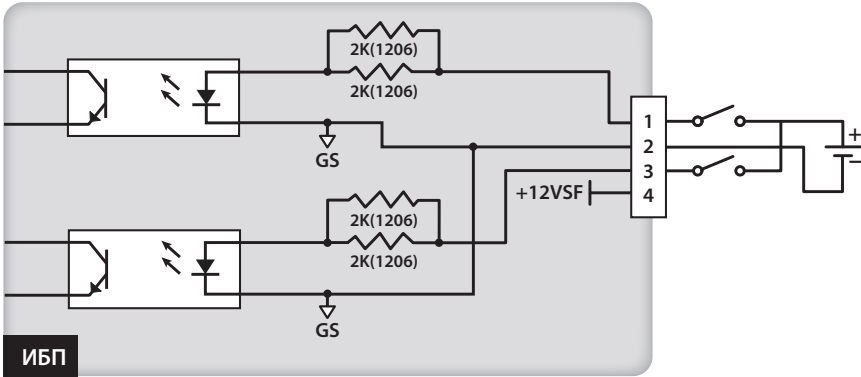
Рис. 5-8. Входы с сухими контактами, конфигурация II
