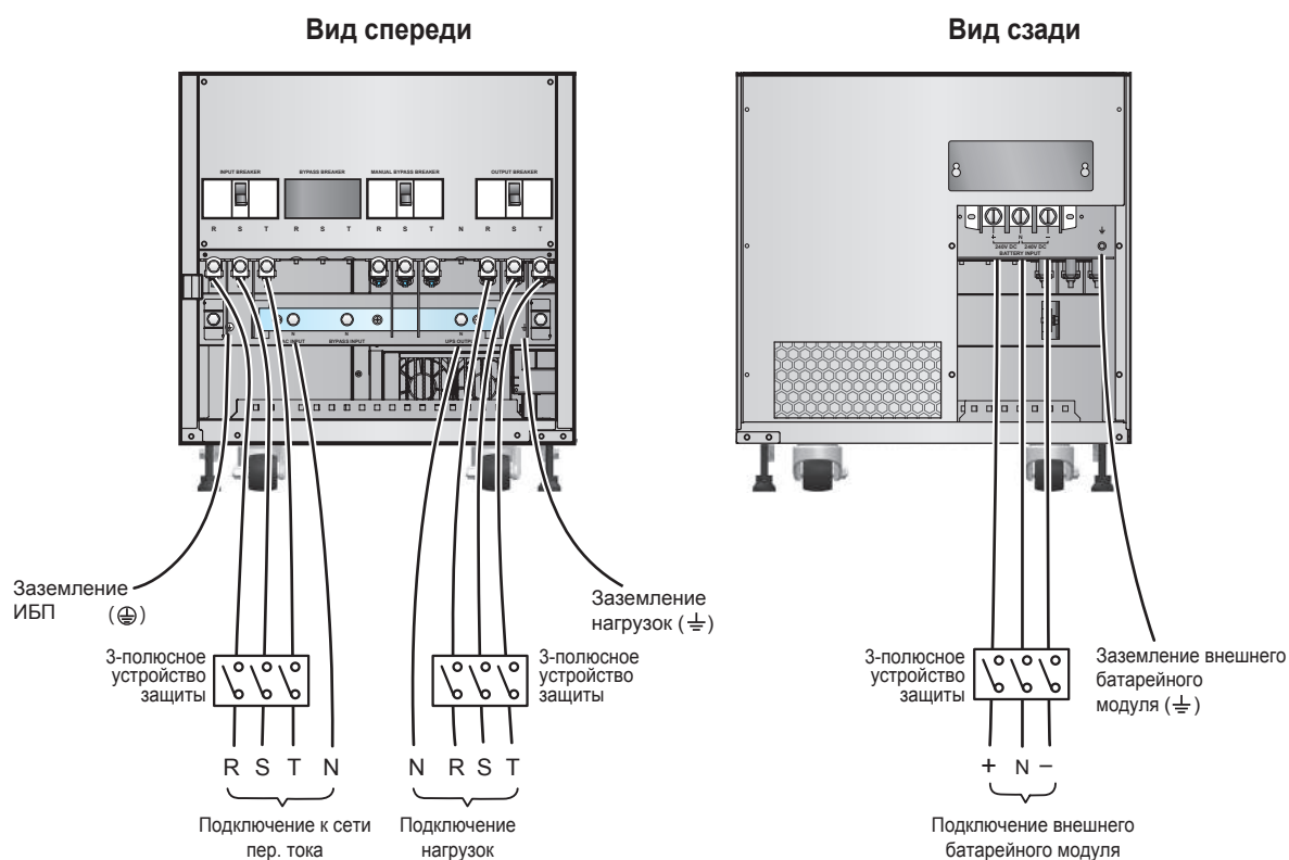
Рис. 6-10. Схема подключения одиночного ИБП 80 кВА в конфигурации с одним входом
