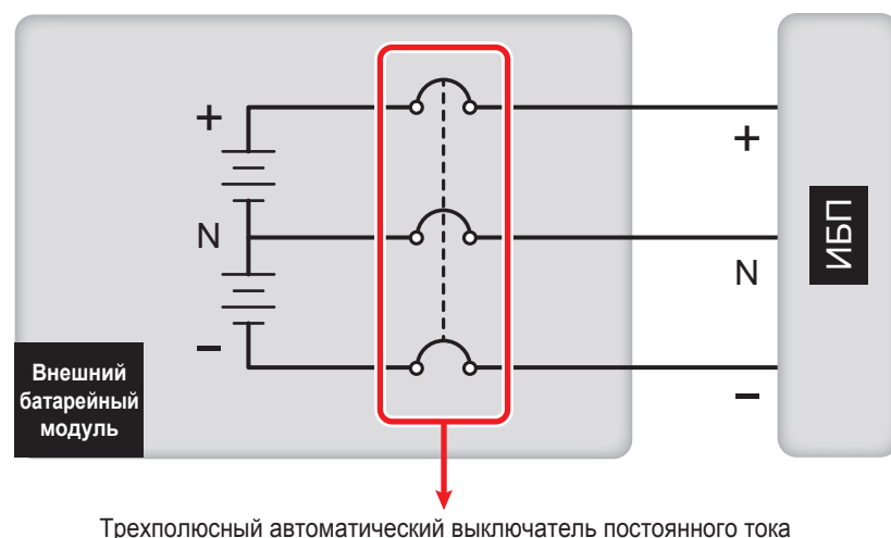
Рис. 6-20. Установка трехполюсного автоматического выключателя постоянного тока
