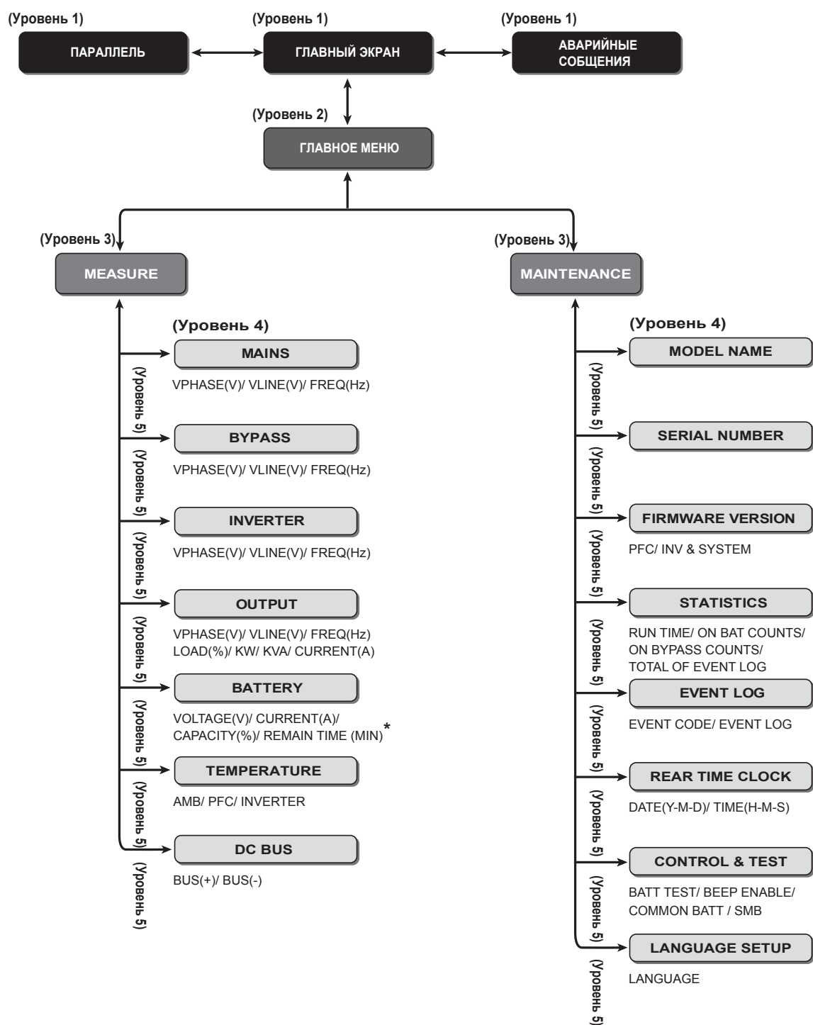
Рис. 8-1. Структура экранных меню
