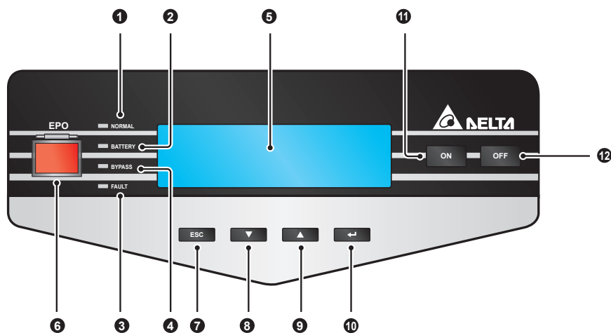
Рис. 3-4. Панель управления
