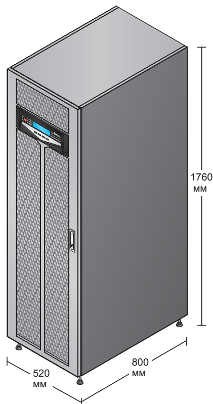
Рис. 3-2. Внешний вид и размеры ИБП 100/120 кВА
