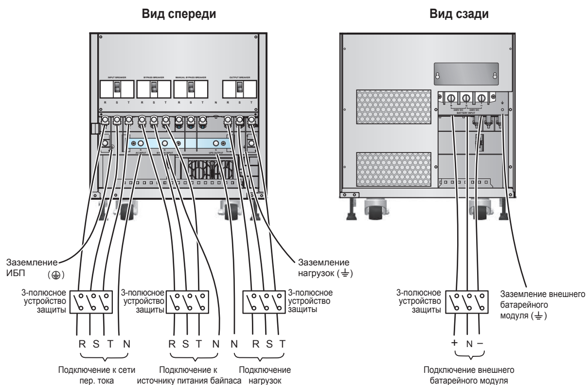
Рис. 6-14. Схема подключения одиночного ИБП 100/120 кВА в конфигурации с двумя входами
