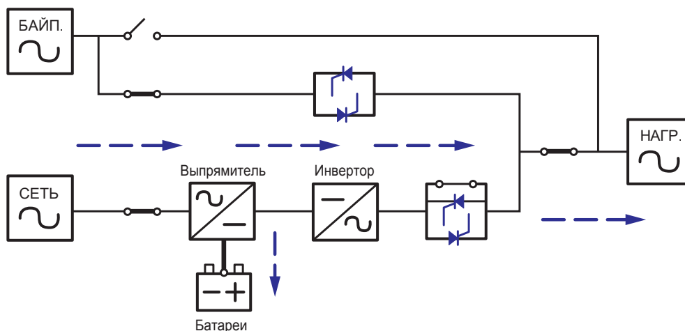
Рис. 4-1. Передача электроэнергии через ИБП в режиме готовности
