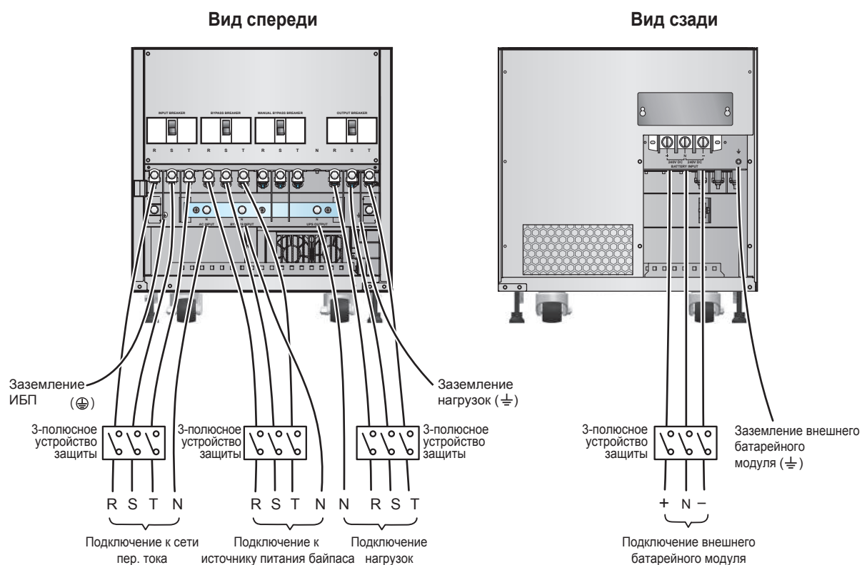
Рис. 6-13. Схема подключения одиночного ИБП 80 кВА в конфигурации с двумя входами
