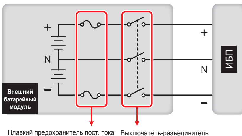
Рис. 6-18. Установка выключателя-разъединителя последовательно с плавким предохранителем постоянного тока
