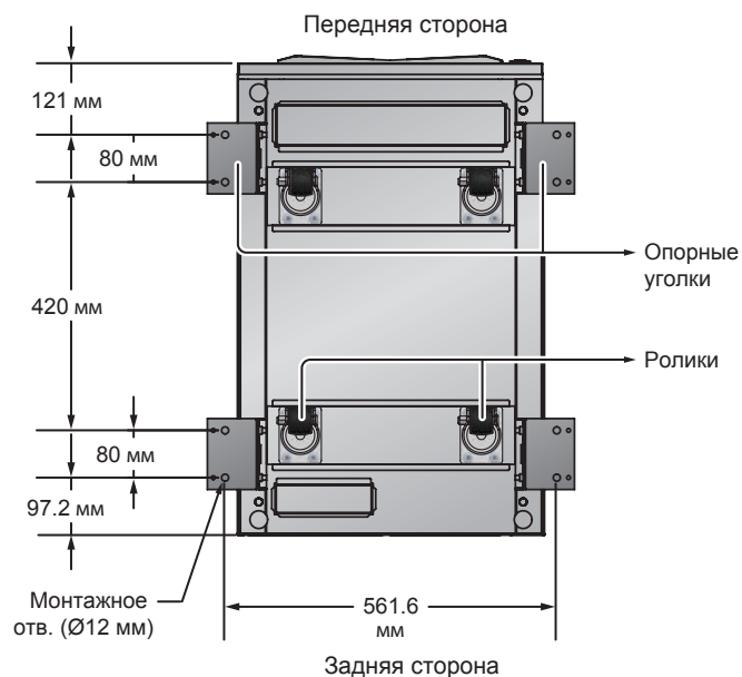
Рис. 6-3. Расположение монтажных отверстий
