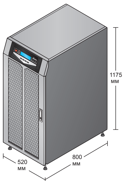
Рис. 3-1. Внешний вид и размеры ИБП 60/80 кВА
